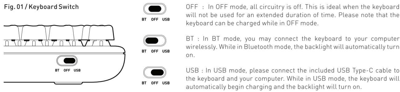
Fig. 01 / Keyboard Switch
